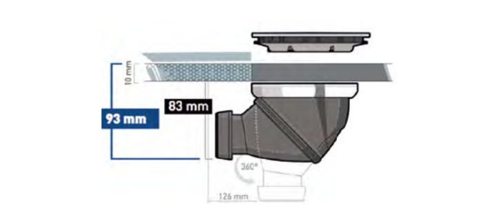
Трап «ВЕНЕЦИЯ МИНИ ДЖЕЙМС» Floor drain VENISIO MINI JAMES
